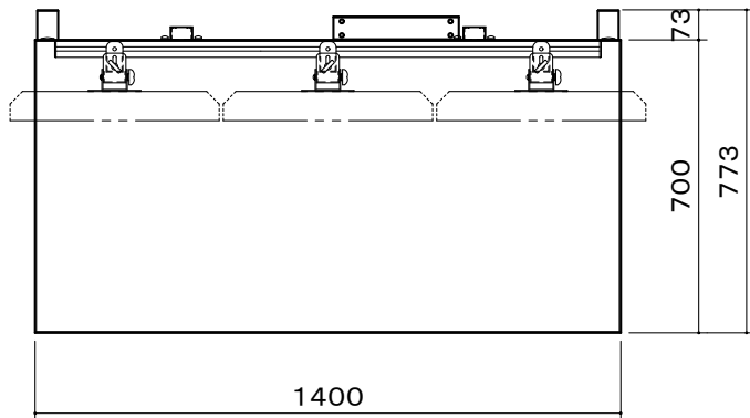
A寸法 ディスプレイ取付金具中心最大W:625
