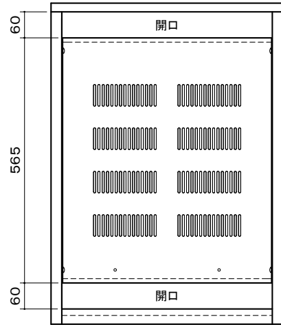
背面図
