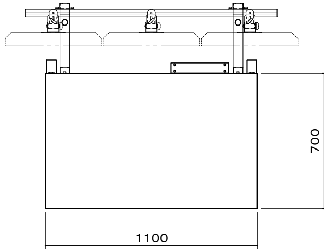
A寸法 ディスプレイ取付金具中心最大W:625
