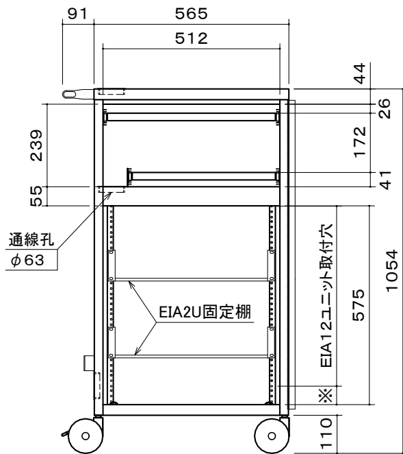
正面開扉時
